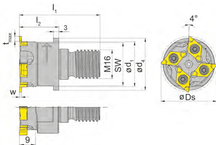
図 = 右勝手バージョン Picture = right hand cutting version
